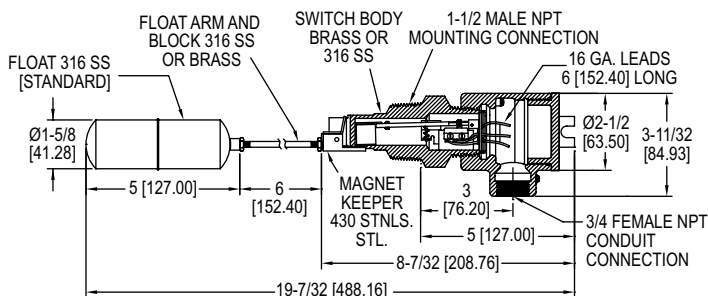
UL/CSA unit
